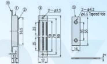
DC-MGCBN2
