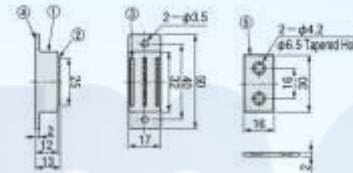
DC-MGCBN1
